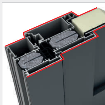
Intérieur et à l'extérieur profilé
